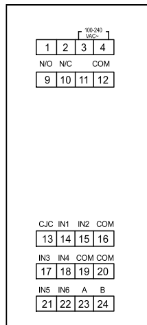
E7 接线图
