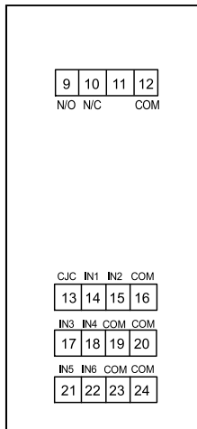
D7 接线图
